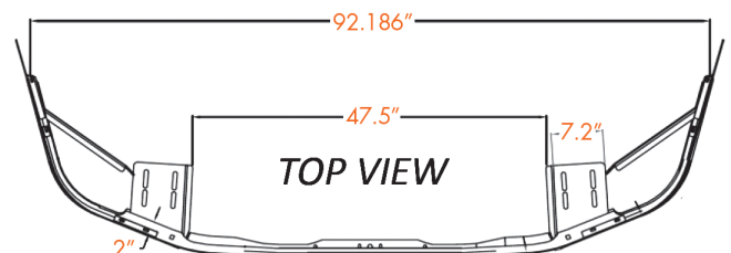
CY-0010-15X Tow pins
